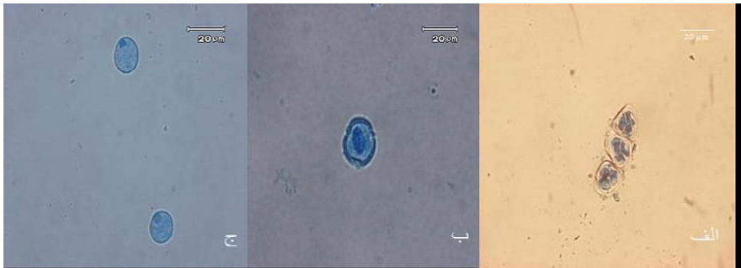
شکل ۱- مراحل نمو میکروسپور در گل محمدی (اکوتیپ کاشان) الف- مرحله تتراد، ب- مرحله تک هسته‌ای میانی، ج- مرحله آخر تک هسته‌ای
