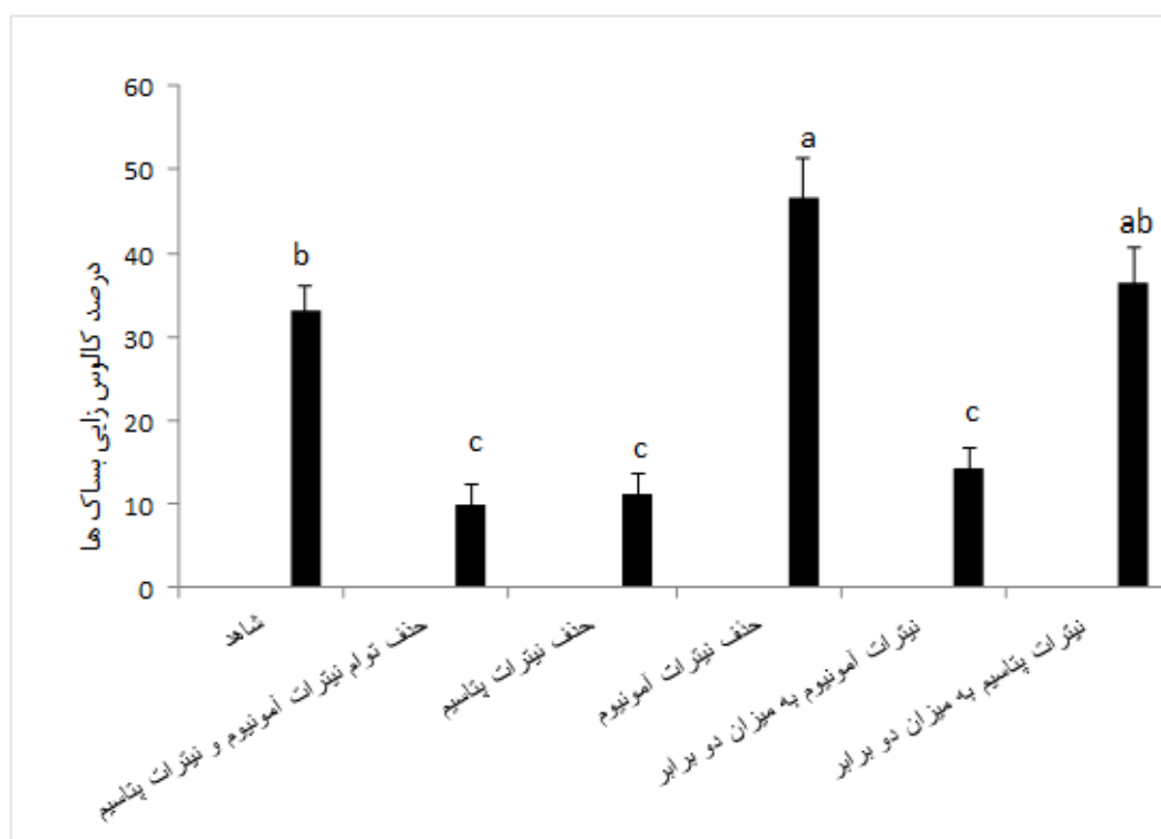
شکل ۷- مقایسه میانگین اثر نسبت نیترات آمونیوم به نیترات پتاسیم برای صفت درصد کالوس زایی بساک‌ها در دو اکوتیپ گل محمدی و رز مینیاتوری
