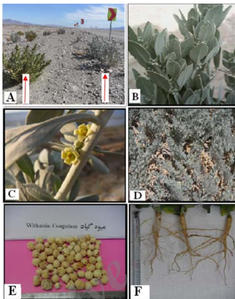
شکل ۲- گونه W. coagulans در زویشگاه سراوان
