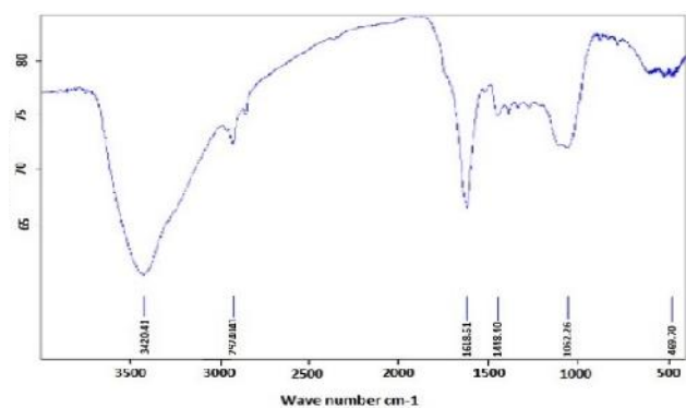
شکل ۱- طیف FT-IR نانوذره آهن
