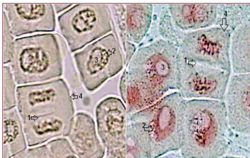
شکل ۴- نمایش مراحل اینترفاز و تروفاز یاخته‌های مریستم نوک ریشه پیاز خوراکی رنگ شده با استوکارمن (راست)
