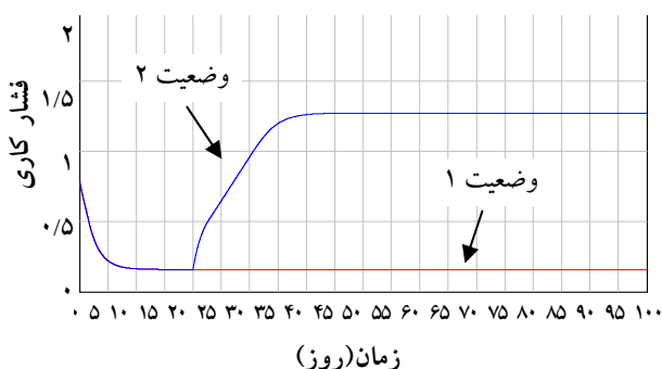
شکل ۹: فشار کاری
