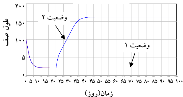
شکل ۸: طول صف با فرض تغییر در نرخ ورود مشتریان
