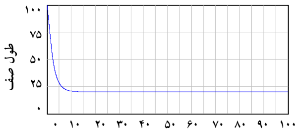
شکل ۴: طول صف زمان (روز)
