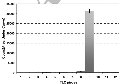
شکل ۴- رادیوکروماتوگرام محلول نهایی پس از عبور از Sep- \text{C}_{18} Pak بر اساس پیک ۱۱ keV
