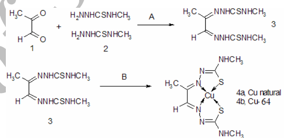
شکل ۲- نمودار شمایی از روش تولید ترکیبات PTSM (3) و Cu-PTSM (4)
