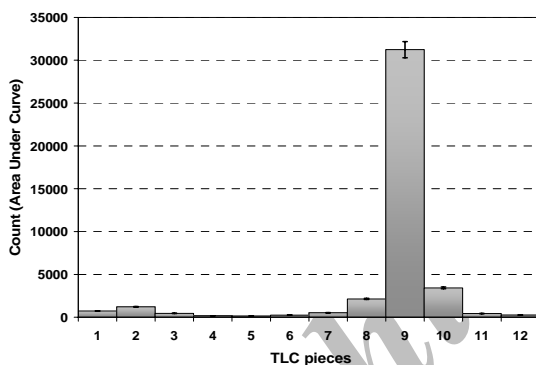
شکل ۳- رادیوکروماتوگرام محلول نشاندار شده قبل از عبور از \text{C}_{18} Sep-Pak بر اساس پیک ۱۱ keV
