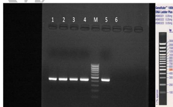
شکل ۳: PCR F1-390 \beta with Pfu DNA Polymerase
