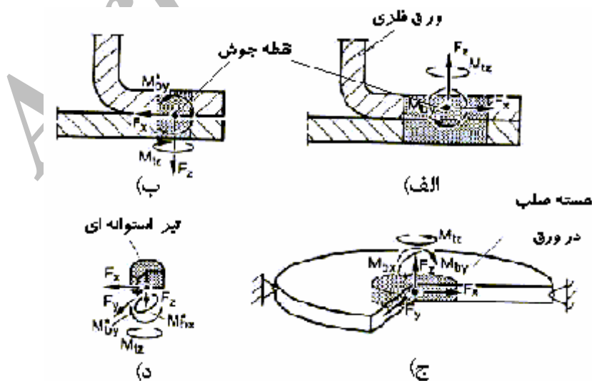
شکل ۱- الف) نیروها و ممان‌های وارد بر نقطه جوش، ب) نیروها و ممان‌های وارد بر ورق در صفحه مشترک دو ورق ج) مدل ساده شده نیروها و ممان‌های وارد بر نقطه جوش، د) مدل ساده شده نیروها و ممان‌های وارد بر ورق در صفحه مشترک دو ورق [۱]
