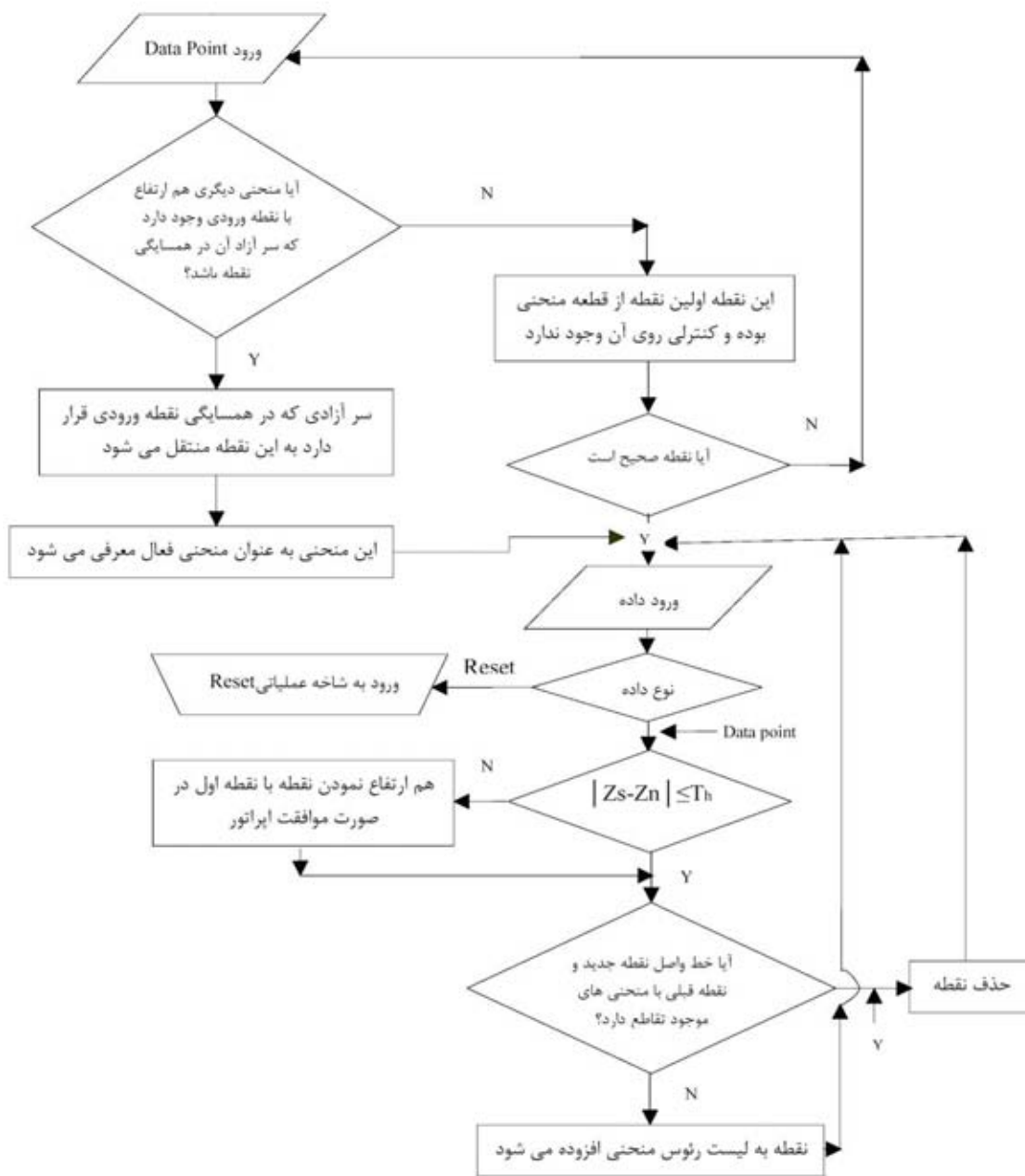
شکل ۵- فلوجارت مربوط به عملکرد سیستم OCBPS در مقابل دریافت Data Point
