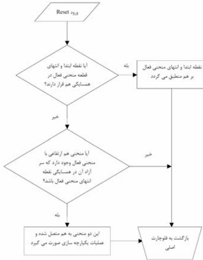
شکل ۶- فلوجارت مربوط به عملکرد سیستم در مقابل دریافت Reset
