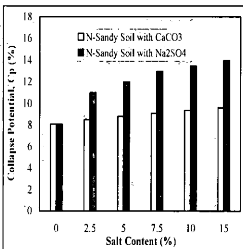
شکل ۵- مقایسه تغییرات پتانسیل رمبندگی ماسه ناشی از حضور افزودنی‌های سولفات سدیم و کربنات کلسیم
