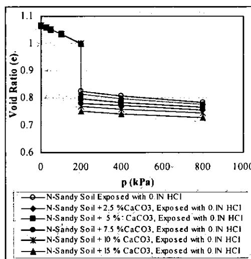
شکل ۸- تغییرات قابلیت رهمندگی نمونه‌های ماسه‌ای حاوی کربنات کلسیم ناشی از اشباع کردن با محلول ۰/۱ نرمال اسید کلریدریک
