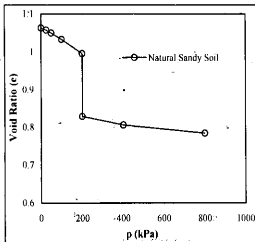
شکل ۲- اندازه‌گیری پتانسیل ریمندگی ماسه مورد آزمایش بر اساس روش ادمتری ساده
