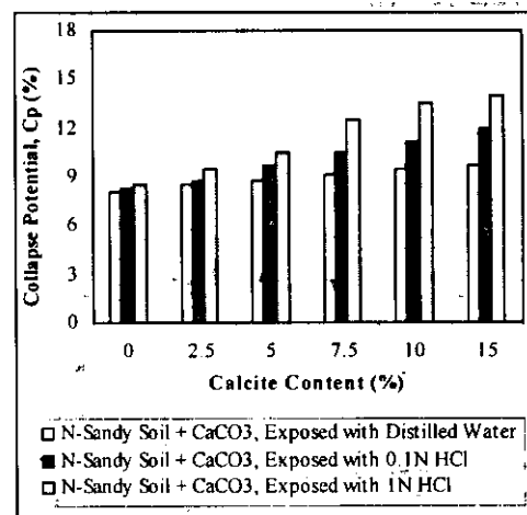
شکل ۱۰- مقایسه تغییرات پتانسیل رمبندگی ماسه ناشی از تغییر مشخصات شیمیایی مایع منفذی و انحلال نمک‌های کربناتی نامحلول
