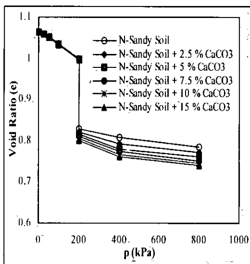
شکل ۴- افزایش اندک قابلیت رمبندگی ماسه ناشی از حضور کربنات کلسیم
