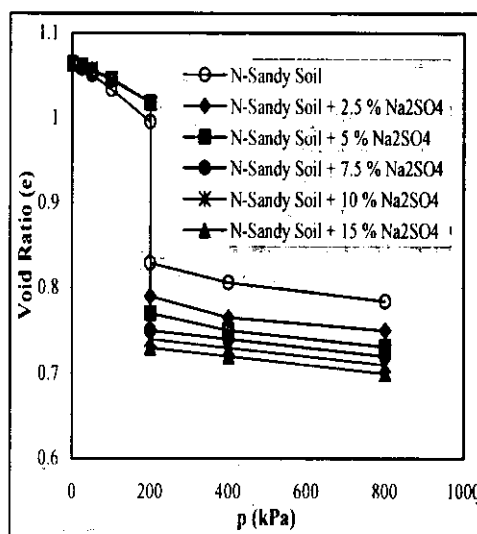
شکل ۳- افزایش قابلیت رمبندگی ماسه ناشی از حضور سولفات سدیم
