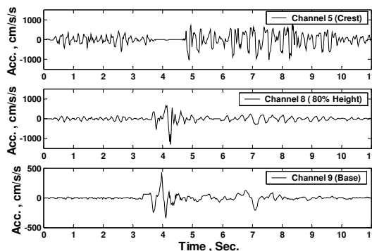
شکل ۳- شتاب نگاشت‌های ثبت شده در کانال ۹، ۸ و ۵
