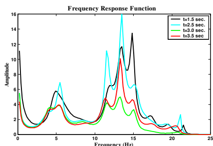
شکل ۱۵- تابع پاسخ فرکانسی در زمان ۳/۵ و ۳، ۲/۵ و ۱/۵ ثانیه
