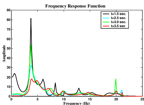
شکل ۱۳- تابع پاسخ فرکانسی در زمان ۳/۵ و ۳، ۲/۵ و ۱/۵ ثانیه
