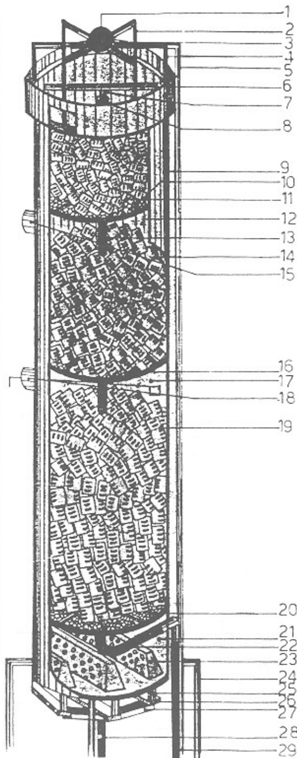
شکل ۲- برش طولی پایلوت
