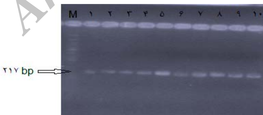
شکل ۱- الکتروفورز ۲ درصد بر روی ژل آگار از محصول PCR و تکثیر قطعه ۲۱۷ bp از ژن prf A
