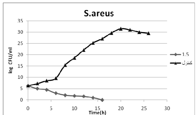
نمودار ۳: اثرات غلظت ۱/۵٪ TiO_2 روی باکتری استافیلوکوکوس ارئوس ( P < 0.05 )
