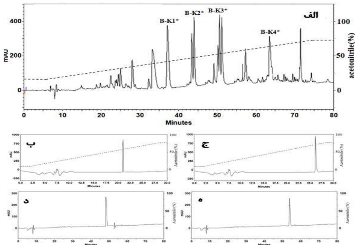
شکل ۱: خالص سازی پپتیدهای ضد میکروبی از ترشحات پوستی وزغ کوبیری بومی یزد توسط کروماتوگرافی RP-HPLC و ستون C18.
