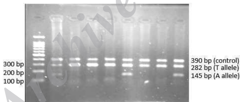
شکل ۲: نمونه‌ای از تعیین ژنوتیپ نشانگر rs1800624 توسط تکنیک Tetra-primer ARMS PCR مربوط به ۸ فرد (طول محصولات PCR در سمت راست شکل قابل مشاهده می‌باشد).
