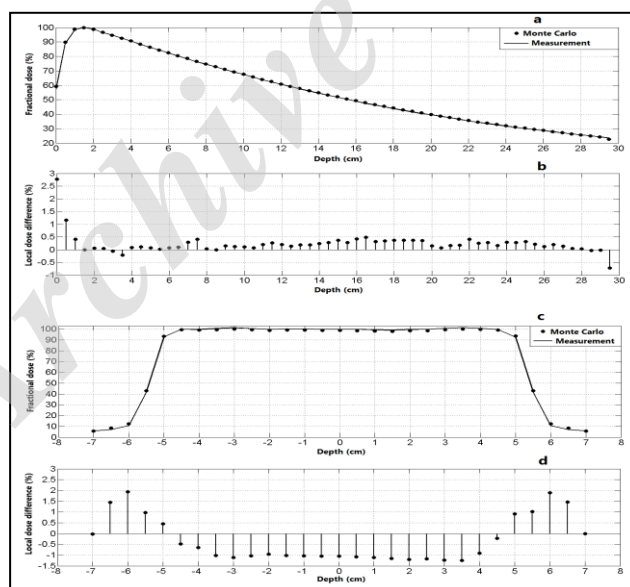
نمودار ۱: مقایسه روش مونت کارلو استفاده شده و نتایج اندازه‌گیری‌های تجربی در اندازه میدان باز 10 \times 10 cm 2 در فانتوم آب در SSD=100 cm برای انرژی فوتون ۶MV (A) محاسبات دوز عمقی در راستای محور مرکزی تابش، (b) اختلاف دوز وابستگی‌های PDD بین روش مونت کارلو و اندازه‌گیری‌های تجربی، (c) محاسبات دوز در راستای محور مرکزی X در عمق ۵cm فانتوم آب، (d) اختلاف دوز وابستگی‌های منحنی پروفایل دوز بین محاسبات مونت کارلو و اندازه‌گیری‌های تجربی. مقدار میانگین عدم قطعیت برای محاسبات مونت کارلو نسبت دوز عمقی و پروفایل دوز به ترتیب \pm 0.16\% و \pm 0.16\% بود.
