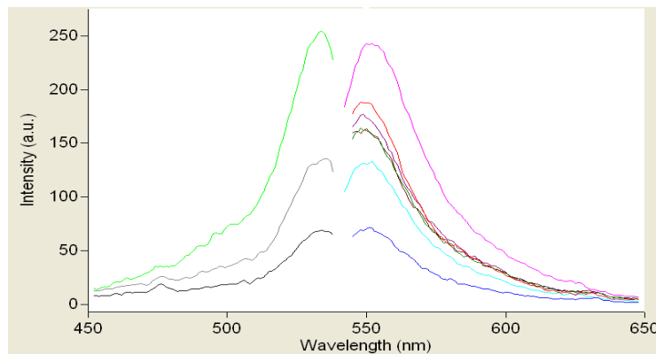
شکل ۱: نمودار طول موجهای ماکزیمم تحریک (۵۳۲ nm ) و تابش (۵۴۳ nm ) کمپلکس فلورسنت حاصل از مالون دی آلدیید در طیف سنجی فلورسانس
