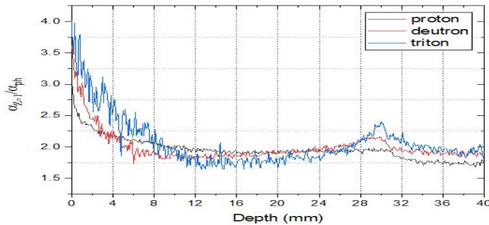
شکل ۲: تغییرات \alpha_{Z=1}/\alpha_{ph} برحسب عمق در فانتوم برای سه یون با Z=1 در رده سلولی B16
