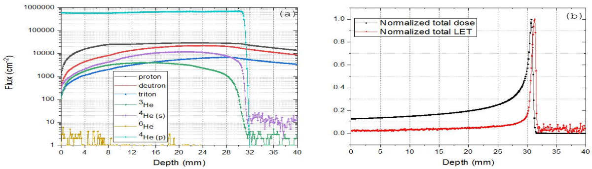
شکل ۱: (الف) شار ذرات تولید شده در میدان تابش برحسب عمق در فانتوم. برای {}^4\text{He} ، علامت s و p، به ترتیب برای یون های اولیه و ثانویه می باشد. (ب) تغییرات دز فیزیکی و LET کل ذرات بر حسب عمق در فانتوم.
