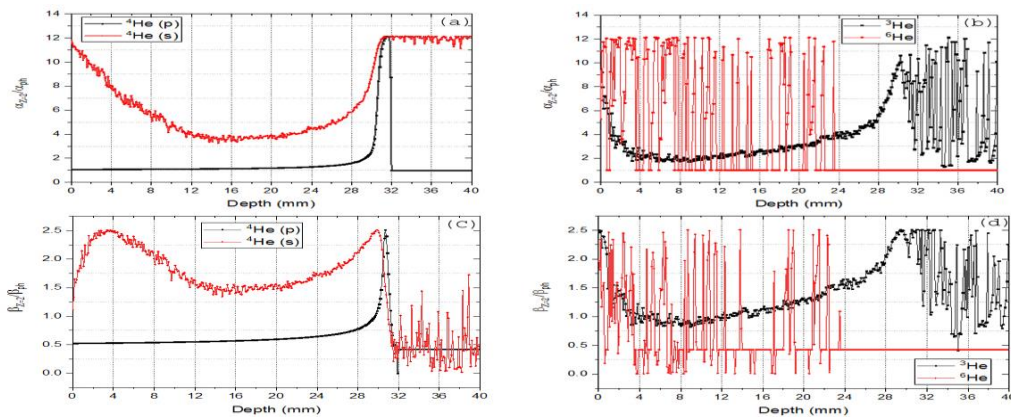
شکل ۳: تغییرات \beta_{Z=2}/\beta_{ph} و \alpha_{Z=2}/\alpha_{ph} برحسب عمق در فانتوم برای چهار نوع یون با Z=2 در رده سلولی B16. برای {}^4\text{He} ، علامت s و p، به ترتیب برای یون های اولیه و ثانویه می باشد.
