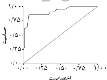
اختصاصیت حساسیت نمودار ۱: منحنی راک برای تعیین نقطه برش مناسب در تشخیص پلورال افیوژن ناشی از سل بوسیله ADA مایع پلور
