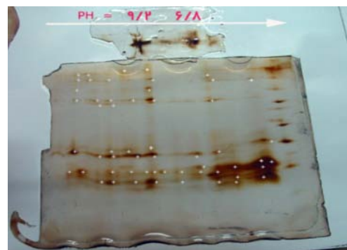
تصویر ۴) ژل الکتروفورز دو بعدی، الگوی پپتیدهای زهر عقرب دوره
