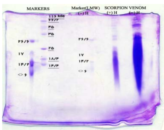
تصویر ۲) مقایسه تأثیر حرارت بر نمونه در ژل SDS-PAGE ستون ها از سمت چپ به راست: ۱- مارکر Fermentas-low molecular weight SM 3410 ۲- مارکر molecular weight ۳- نمونه به مدت ۵ دقیقه در آب جوش حرارت داده شد ۴- نمونه بدون حرارت
