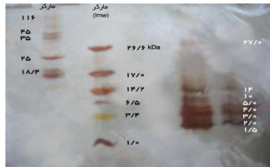
تصویر ۳) مقایسه الگوی پپتیدهای زهر عقرب‌های دوره و کراسیکودا توسط ژل تریسین با غلظت ۱۶/۵ درصد
