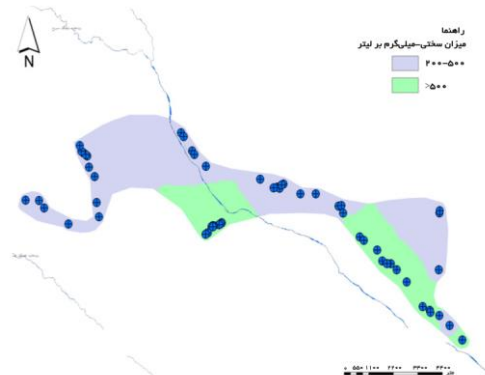
شکل ۳) توزیع مکانی غلظت سختی منطقه مورد مطالعه برحسب میلی‌گرم بر لیتر کرنات کلسیم
