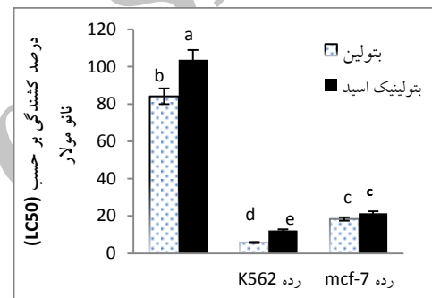
نمودار ۲) مقایسه تأثیر تیمارهای عصاره گیاهی (بتولین و بتولینیک اسید) بر سلول های سرطانی K562، MCF-7 و آرتیمیا ارومیانا با استفاده از آزمون رنگ تریپان بلو و تست میگوی آب شور. هر ستون نشان دهنده میانگین داده ها ± انحراف استاندارد. ستون ها دارای حداقل یک حرف مشترک با آزمون دانکن در سطح احتمال ۵ درصد تفاوت معنی داری ندارند.
