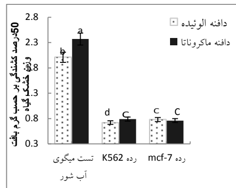
نمودار ۱) مقایسه تأثیر تیمارهای عصاره گیاهی (دافنه الوئیده و دافنه ماکروناتا) بر سلول های سرطانی K562، MCF-7 و آرتیمیا ارومیانا با استفاده از آزمون رنگ تریپان بلو و تست میگوی آب شور. هر ستون نشان دهنده میانگین داده ها ± انحراف استاندارد. ستون ها دارای حداقل یک حرف مشترک با آزمون دانکن در سطح احتمال ۵ درصد تفاوت معنی داری ندارند.
