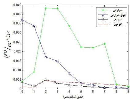
شکل ۹) دوز مؤثر مؤلفه‌های نوترون و اشعه گاما (فوتون) در عمق‌های مختلف فانتوم فاقد تومور. غلظت بور در مغز 40 \text{ ppm} است.
