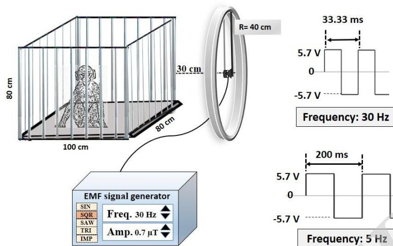
شکل ۲) نمای شماتیک از پالس مربعی ایجاد شده توسط یک سیگنال ژنراتور و انتقال به یک آنتن دایره‌ای شکل به شعاع ۴۰ سانتی‌متر. قفس حاوی میمون در فاصله ۳۰ سانتی‌متری از قفس قرار گرفته و در معرض پرتو قرار می‌گیرد.
