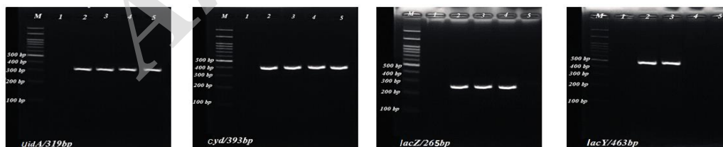
شکل ۱) اختصاصیت پرایمرهای تشخیصی، LacY ، Cyd ، Uida ، LacZ در سویه‌های کنترل. M: مارکر ملکولی DM2300. ۱: کنترل منفی، ۲: انتروهومورازیک اشرشیا کلی (G4S42)، ۳: انتروهومورازیک اشرشیا کلی (G4S45)، ۴: شیگلا سونشی (ATCC9290)، ۵: شیگلا فلکسنری (ATCC12022).
