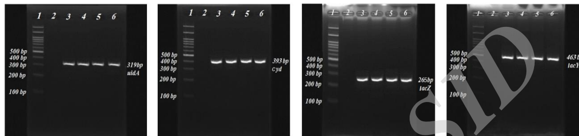
شکل ۲) الکتروفورز محصول PCR با پرایمرهای LacY و Cyd, UidA, LacZ برای تشخیص جدایه‌های محیطی اشرشیا کلی. چاهک‌های شماره ۱: مارکر DM 2300. ۲: کنترل منفی، ۳: اترو همورازیک اشرشیا کلی (G4S42) به عنوان کنترل مثبت، ۴: جدایه محیطی اشرشیا کلی ۵: جدایه محیطی اشرشیا کلی ۱۰۰: جدایه محیطی اشرشیا کلی ۲۳۰. جدایه‌های محیطی اشرشیا کلی همانند سویه کنترل مثبت دارای پاسخ مثبت PCR برای تمامی پرایمرهای تشخیصی هستند.
