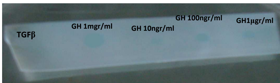
شکل ۱. نتایج Dot blot آنتی‌بادی پلی‌کلونال بر ضد هورمون رشد که در آن TGFβ به عنوان کنترل منفی و هورمون رشد در رقت‌های مختلف استفاده شد.
