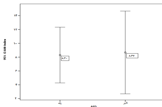
شکل ۳. میانگین و فاصله‌ی اطمینان AHI (Apnea hypopnea index) بر حسب AED
