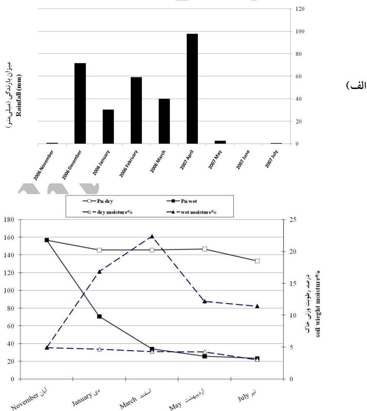
شکل ۴. الف: میزان بارندگی در طول اجرای آزمایش؛ ب: تغییرات جمعیت Pratylenchus neglectus در خاک آلوده بدون حضور میزبان در شرایط میکروپلات در دو حالت بدون بارندگی و با بارندگی.
