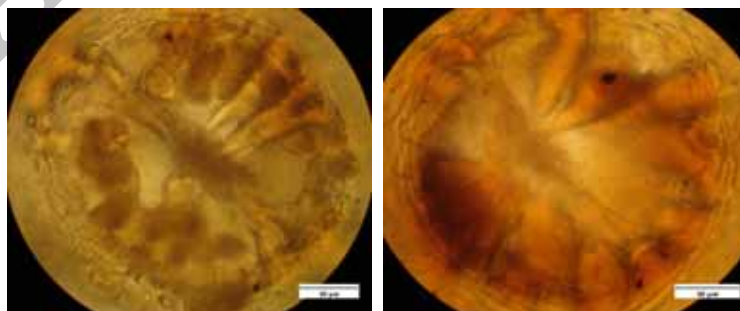
شکل ۵. مخروط انتهایی بدن با باندهای کوتیکولی ناحیه واژن بلند و تعداد زیاد برجستگی‌های گره مانند
