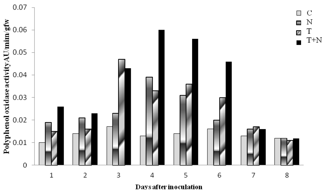
شکل ۳. فعالیت آنزیم پلی فنل اکسیداز در برگ گوجه فرنگی در اثر مایه زنی با Trichoderma harzianum i25 و نماتود ریشه گرهی Meloidogyne javanica . اعداد میانگین ۳ تکرار است. T: قارچ T. harzianum i25 ; N: نماتود ریشه گرهی M. javanica ; C: گیاه سالم (شاهد).
