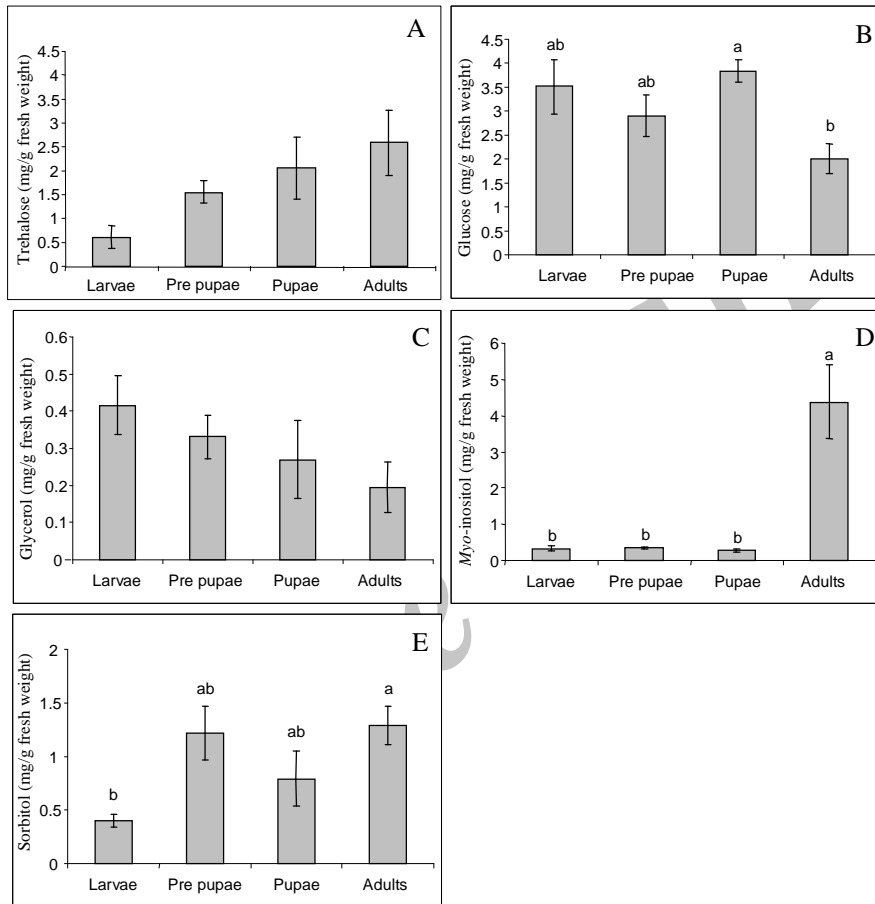
شکل ۴. تغییرات غلظت ترکیبات ضد یخ با وزن مولکولی پایین در مراحل سنی مختلف کرم برگ‌خوار چغندر پرورش‌یافته در آزمایشگاه. A- تری‌هالوز، B- گلوکز، C- گلیسرول، D- مایواینوزیتول و E- سوربیتول. حروف مشابه نشان‌دهنده‌ی عدم وجود اختلاف معنی‌دار در سطح ۵ درصد در آزمون توکی می‌باشد.
