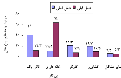
نمودار ۲- توزیع فراوانی نسبی شغل واحدهای پژوهش قبل و بعد از سن بازنشستگی
