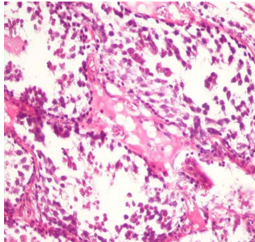
شکل ۱- نمای میکروسکوپی از لوله‌های اسپرم‌ساز گروه تجربی اول (۲۰۰ میلی‌گرم مترونیدازول) به کندی روند اسپرماتوزن و تخلیه برخی لوله‌های اسپرم‌ساز و کاهش سلول‌های لیدیگ و افزایش چربی بین سلولی توجه نمایید (رنگ‌آمیزی H-E و \times 100 )
