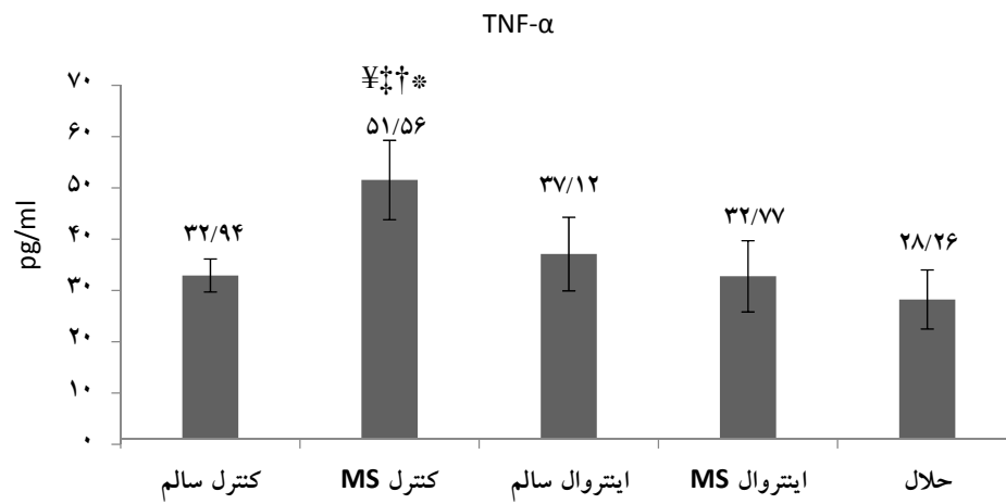
نمودار شماره ۲- میانگین تغییرات TNF- \alpha در گروه‌های مطالعه نشان از معنی داری این شاخص دارد ( P=0/001 ). * تفاوت معنی دار با کنترل سالم ( P=0/001 ) تفاوت معنی دار با ایپتروال سالم ( P=0/01 ), † تفاوت معنی دار با ایپتروال MS ( P=0/001 ) و ‡ تفاوت معنی دار با گروه حلال ( P=0/001 )
