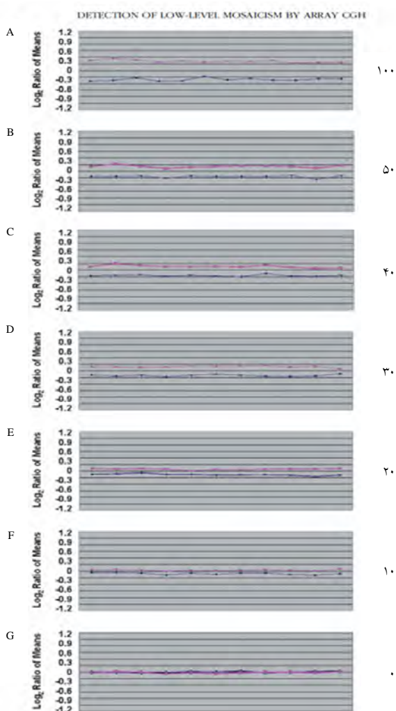
شکل-۲: شناسایی سطوح پایین موزایسم به وسیله آرایه CGH. ۳۱
