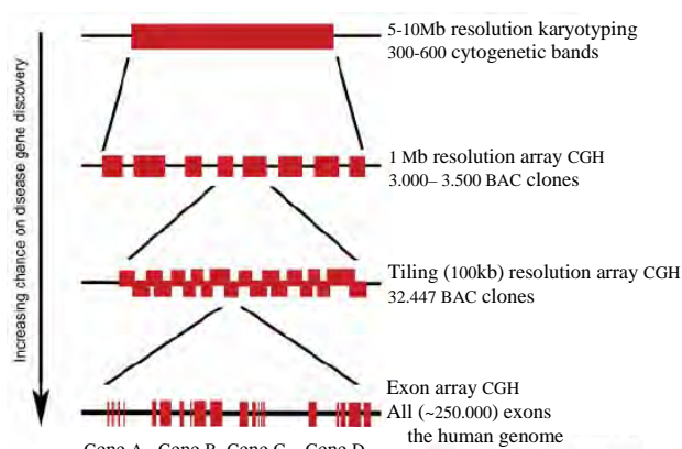
شکل ۳: تاثیر افزایش قدرت تفکیک روش‌های مطالعه ژنوم بر شناسایی ژن‌های درگیر در بیماری‌زایی. ۴۸
