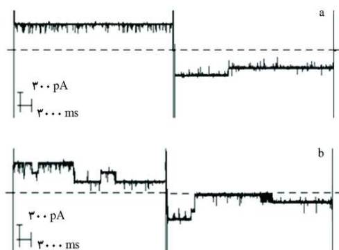
شکل ۲: جریان عبوری از کانال منفرد OmpF در ولتاژ 140 \pm میلی‌ولت، در دمای 20^\circ\text{C} و \text{pH } 7/4 به مدت ۱۰ دقیقه در دو حالت (a) حالت کنترل (وضعیت خاموش گوشی تلفن همراه) (b) تحت تابش امواج گوشی تلفن همراه (وضعیت روشن گوشی)
