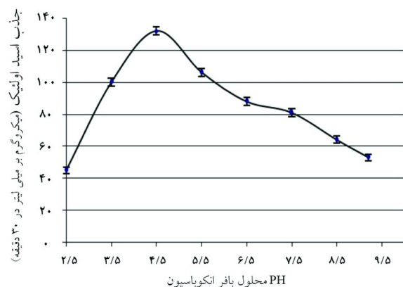
نمودار ۱: اثر pH بر میزان برداشت اسید اولئیک توسط EGS.
