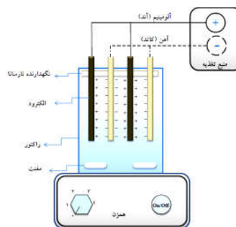
شکل ۱: راکتور الکتروشیمیایی و اتصال تک‌نقطه‌ای موازی الکترودها به منبع تغذیه
