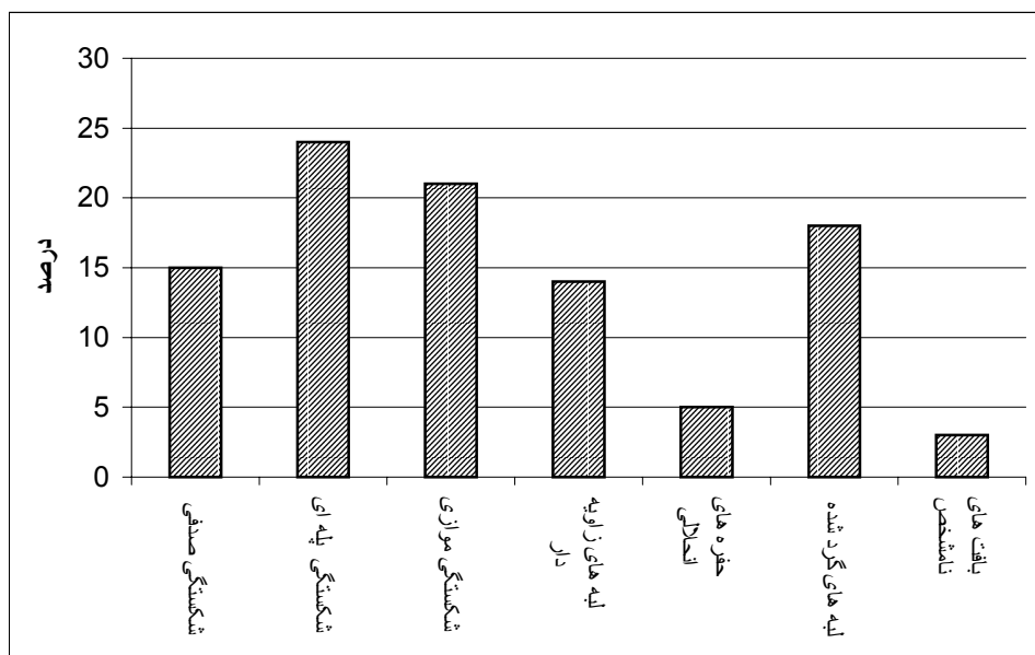
شکل ۵- درصد فراوانی نسبی انواع بافت سطحی در دانه های کوارتز ۱۰۰-۳۰۰ میکرون در رسوبات لس گلستان
