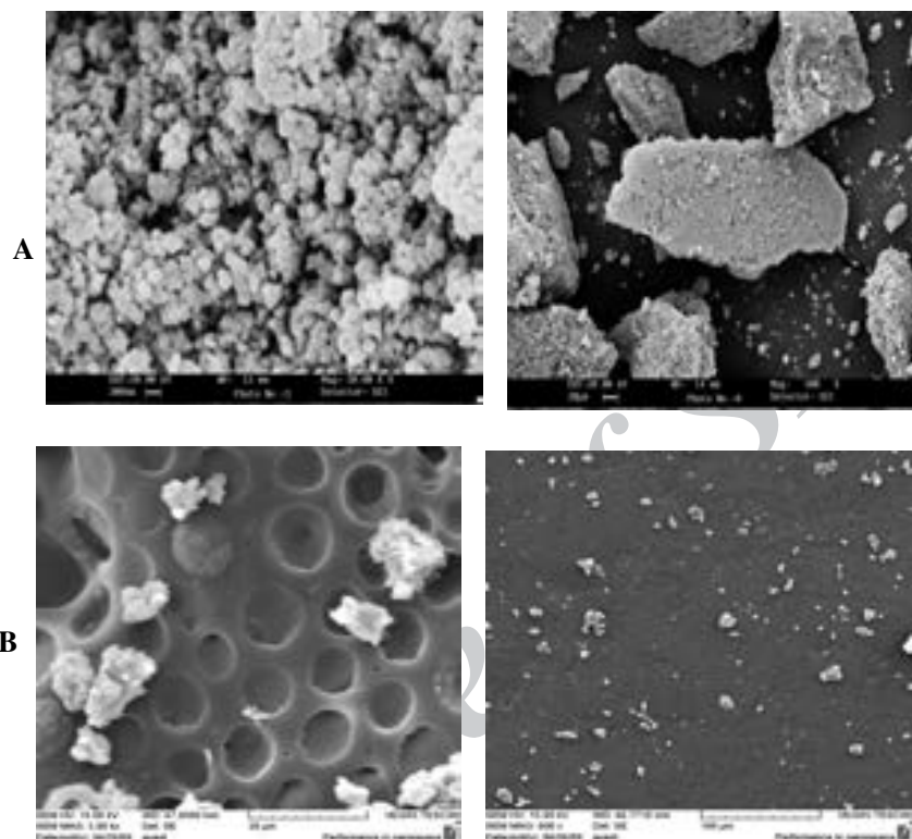
شکل ۳. تصاویر SEM (A) PANI/HCl، (B) نانو کامپوزیت PANI/PSMAC/PSS
