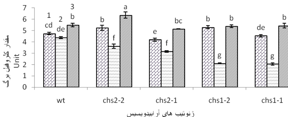
شکل ۳. اثر تیمارهای دمایی پایین روی مقدار کلروفیل کل در گیاهان وحشی و جهش یافته آرابتیوپسیس. ۱: تنش سرما، ۲: تیمار سرما، ۳: شاهد
