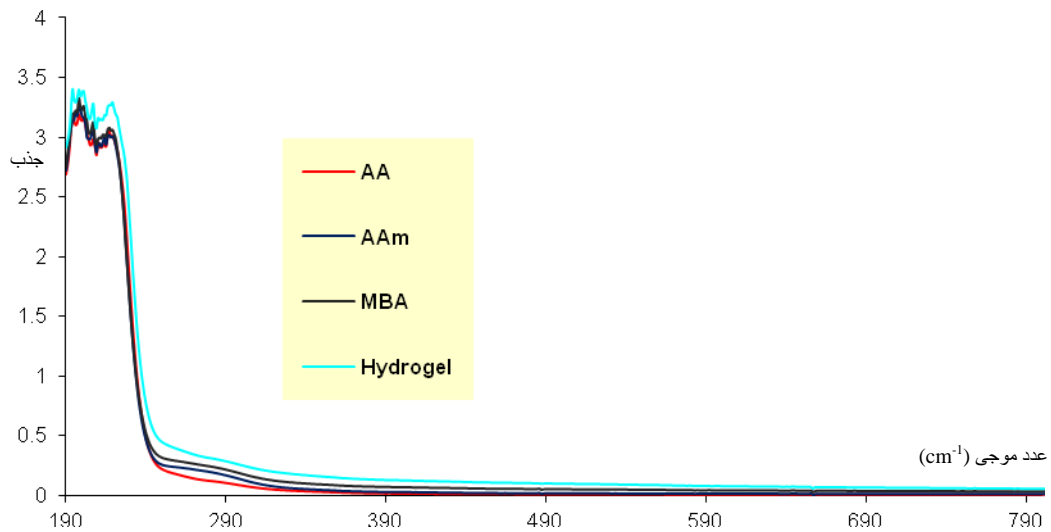
شکل ۶. طیف UV مونومرهای آکریل آمید، آکرلیک اسید، شبکه‌ساز MBA و هیدروژل به دست آمده از آن‌ها
