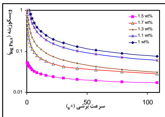
شکل 4: رفتار جریان‌یابی سوسپانسیون در 50 درصد حجمی جامد برای مقادیر مختلف پراکنده‌ساز دولایپیکس ET85.
