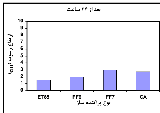
شکل 2: تست رسوب پراکنده‌سازهای مختلف بعد از 24 ساعت.
