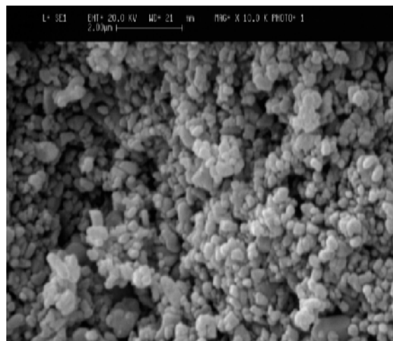
شکل 7: تصویر میکروسکوپ الکترونی روبشی بدنه خام نانوکامپوزیت Al_2O_3/Ag .
