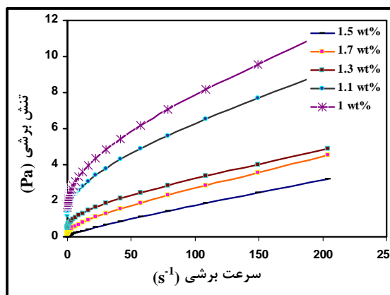
شکل 5: تنش برشی بر حسب سرعت برشی در 50 درصد حجمی جامد برای مقادیر مختلف پراکنده‌ساز دولاپیکس ET85.
