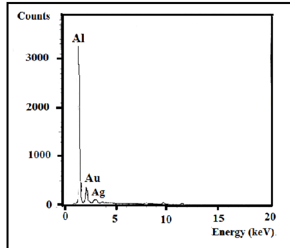
شکل 9: آنالیز EDX نانوکامپوزیت Al_2O_3/Ag .
