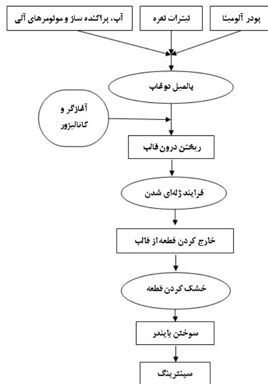
شکل 1: فلوچارت فرآیند ریخته‌گری ژلی نانوکامپوزیت \text{Al}_2\text{O}_3/\text{Ag} .
