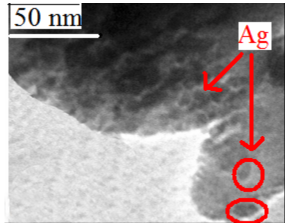
شکل 11: تصویر میکروسکوپ الکترونی عبوری نانوکامپوزیت Al_2O_3/Ag .
