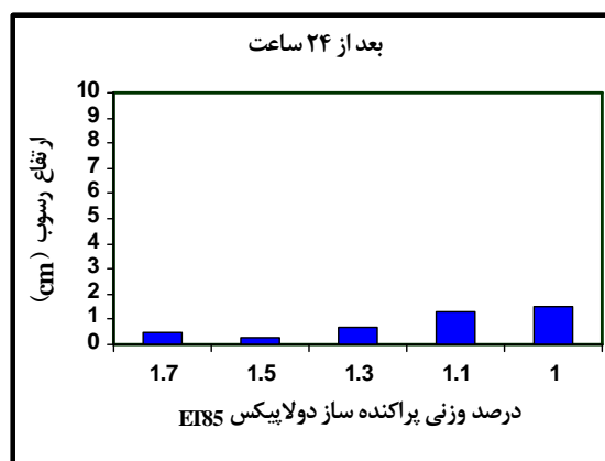
شکل 3: رفتار رسوبی درصدهای مختلف پراکنده‌ساز ET85.
