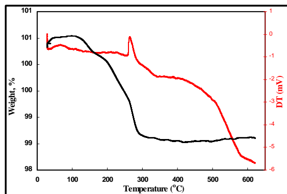
شکل 6: منحنی‌های آنالیز حرارتی (DTA-TG) نانوکامپوزیت \text{Al}_2\text{O}_3/\text{Ag}
