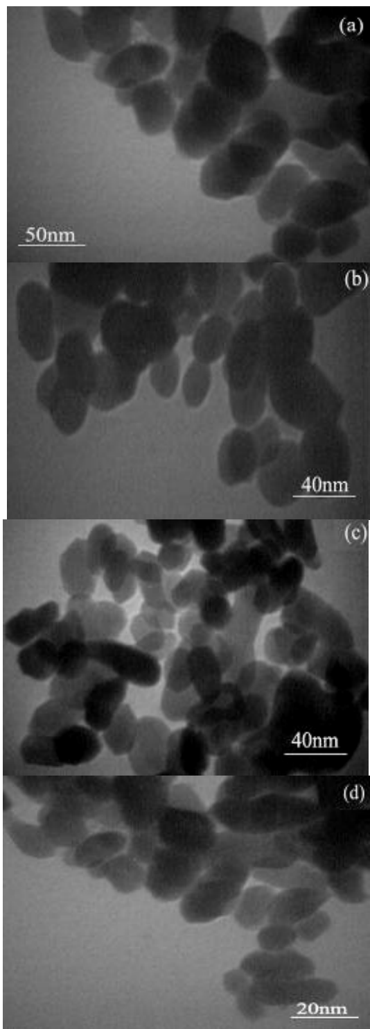
شکل ۲: تصویر میکروسکوپ الکترونی عبوری نانوذرات سنتز شده \gamma\text{-Fe}_2\text{O}_3 در توان‌های اولیه (a) ۲۰ W، (b) ۴۰ W، (c) ۶۰ W و (d) ۱۰۰ W.
