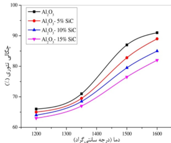
شکل ۴: نمودار چگالی بر حسب دمای سینتر کردن کامپوزیت آلومینا-سیلیکون کاربرد و مقایسه آن با آلومینای خالص.
