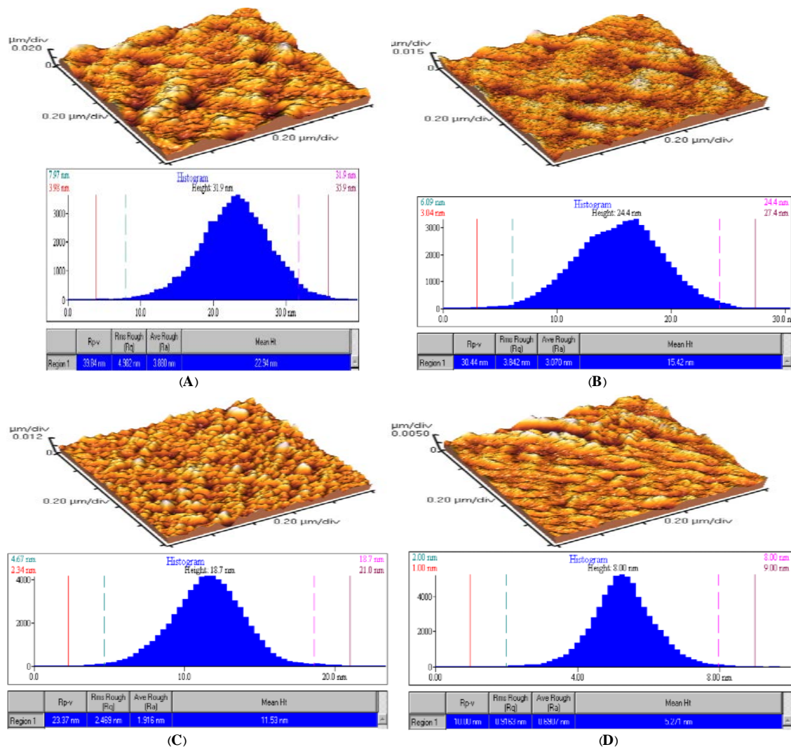
شکل ۳: ریزساختار سطح توسط میکروسکوپ نیروی اتمی (AFM) نمونه‌ها (A) نمونه خالص، (B) (۰/۲۵ N, ۱/۱ Ce - TiO 2 ) (C) (۰/۲۵ N, ۳/۱۰ Ce - TiO 2 ) (D) (۱ N, ۱/۱ Ce - TiO 2 )
