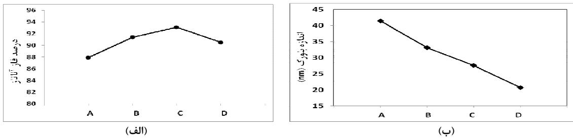
شکل ۲: (الف) روند تغییرات درصد فاز آناز و (ب) روند تغییرات اندازه بلورک‌های نمونه‌های A، B و C و D.
