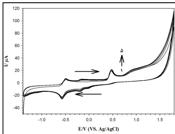
شکل ۱: الکتروپلیمریزاسیون MWCNTs-ARS در سطح الکتروود کربن شیشه در ۱۰/۰ mL بافر فسفاتی با pH=۷/۰ با غلظت ۰/۰۶۷ mol.L -1 حاوی ۶/۰ mg و ۸/۰ mg MWCNTs، سرعت روبش: ۰/۱۰۰ mV.s -1 .
