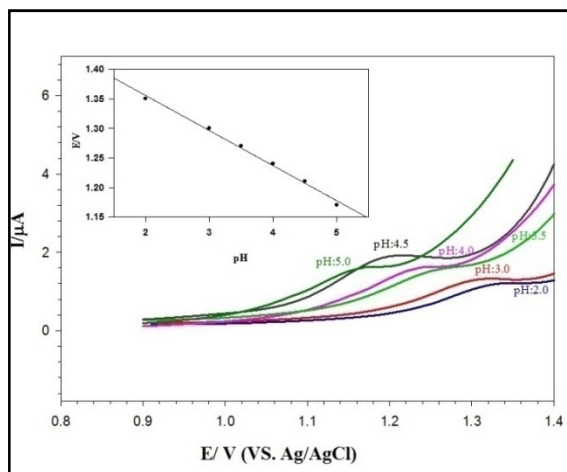
شکل ۵: ولتاموگرام پالس تقاضلی محلول 10/0 \mu\text{mol L}^{-1} جم فیروزیل در سطح MWCNTs-PARS/GCE در محلول بافر فسفاتی با pH های مختلف از ۲٫۰ تا ۵٫۰. سرعت روبش 50 \text{ mV.s}^{-1} ، ارتفاع پالس 70 \text{ mV} ، مدت زمان اعمال پالس 20 \text{ ms} ، تغییرات پتانسیل دماغه اکسایش جم فیروزیل را بر حسب pH نشان می‌دهد.
