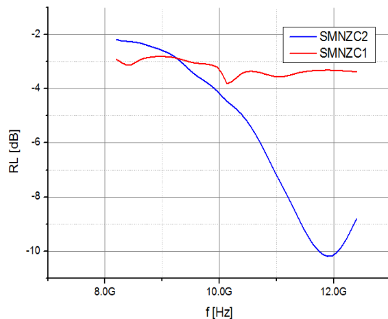
شکل ۱۲: آزمون VNA نمونه های چهار تایی.
