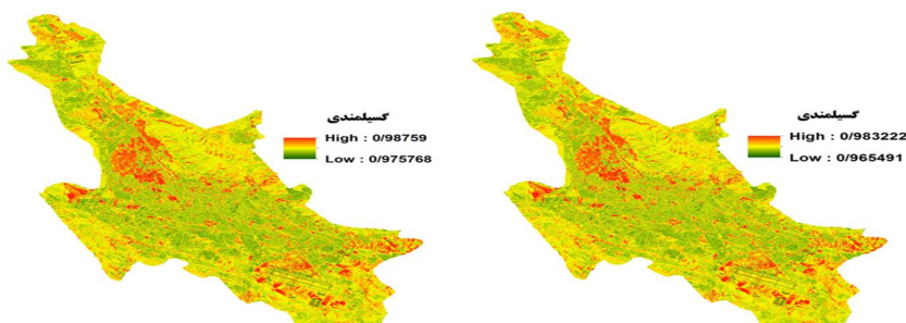
شکل (۹): گسیلمندی حساب شده برای داده زمستان، سمت راست برای باند ۱۳ و سمت چپ برای باند ۱۴
