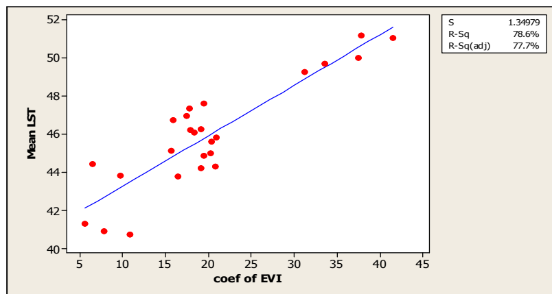
شکل (۱۸): رابطه بین میانگین دمای شهرها و ضریب EVI مربوط به رابطه بین EVI و دمای سطح
