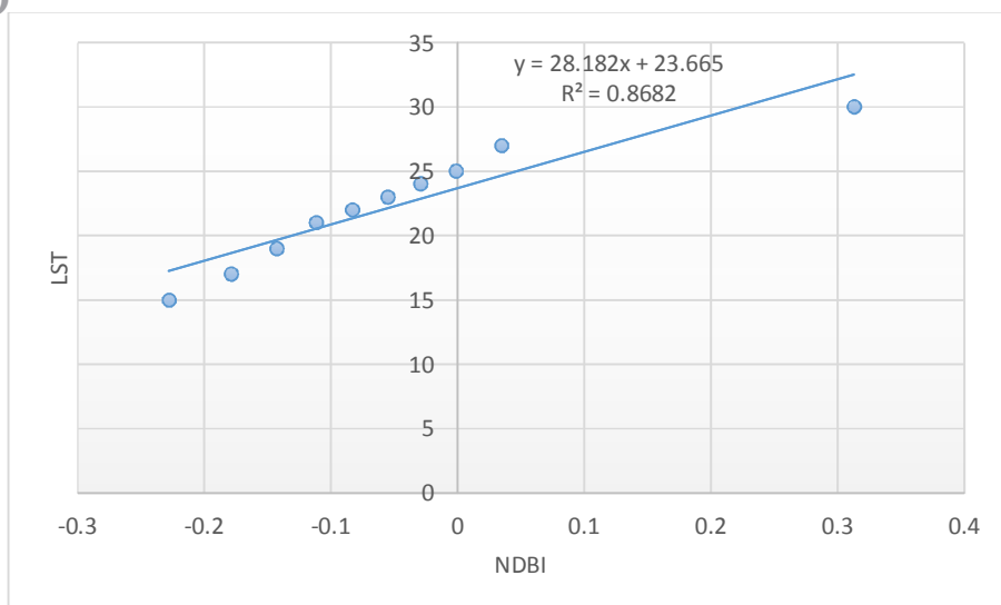
شکل (۲۵): رابطه NDBI و دمای سطح زمین
